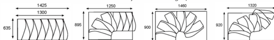
Montážní varianty / assembling options
